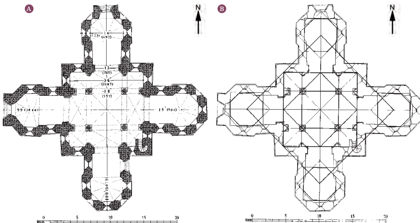
Fig. 4.A-B. Kalundborg, Vor Frue Kirke. Grundplaner med studier af mål, proportioner og geometrisk konstruktion
